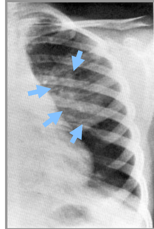
VİRAL PNÖMONİ
