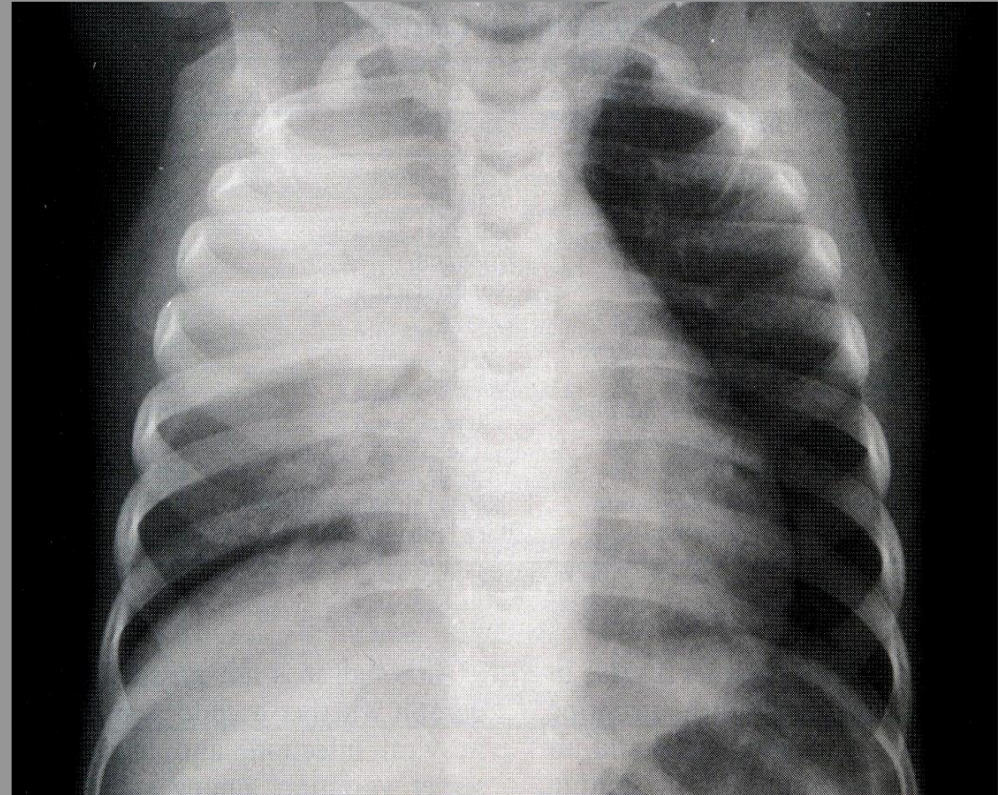
Streptococcus pneumoniae
